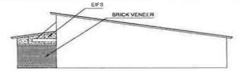
SIDE ELEVATION ——— SCALE: 1/8"=1'-0"
