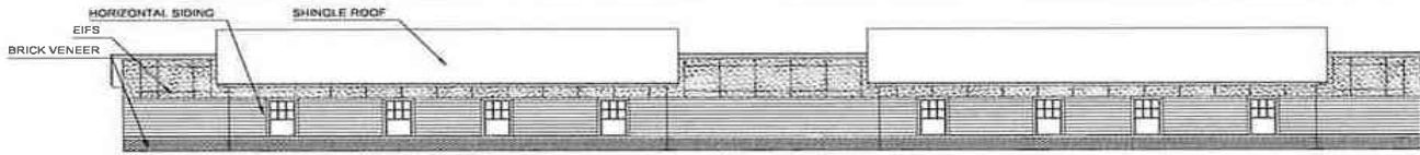
(4) -2BR / (0) -1 BR / (4) -GARAGE REAR ELEVATION ——— SCALE: 1/8"=1'-0"
