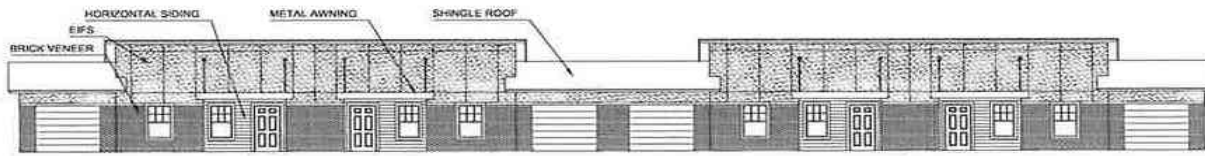
(4) -2BR / (0) -1 BR / (4) -GARAGE FRONT ELEVATION ——— SCALE: 1/8"=1'-0"
